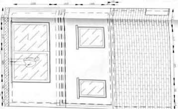
ACHTERGEVEL
